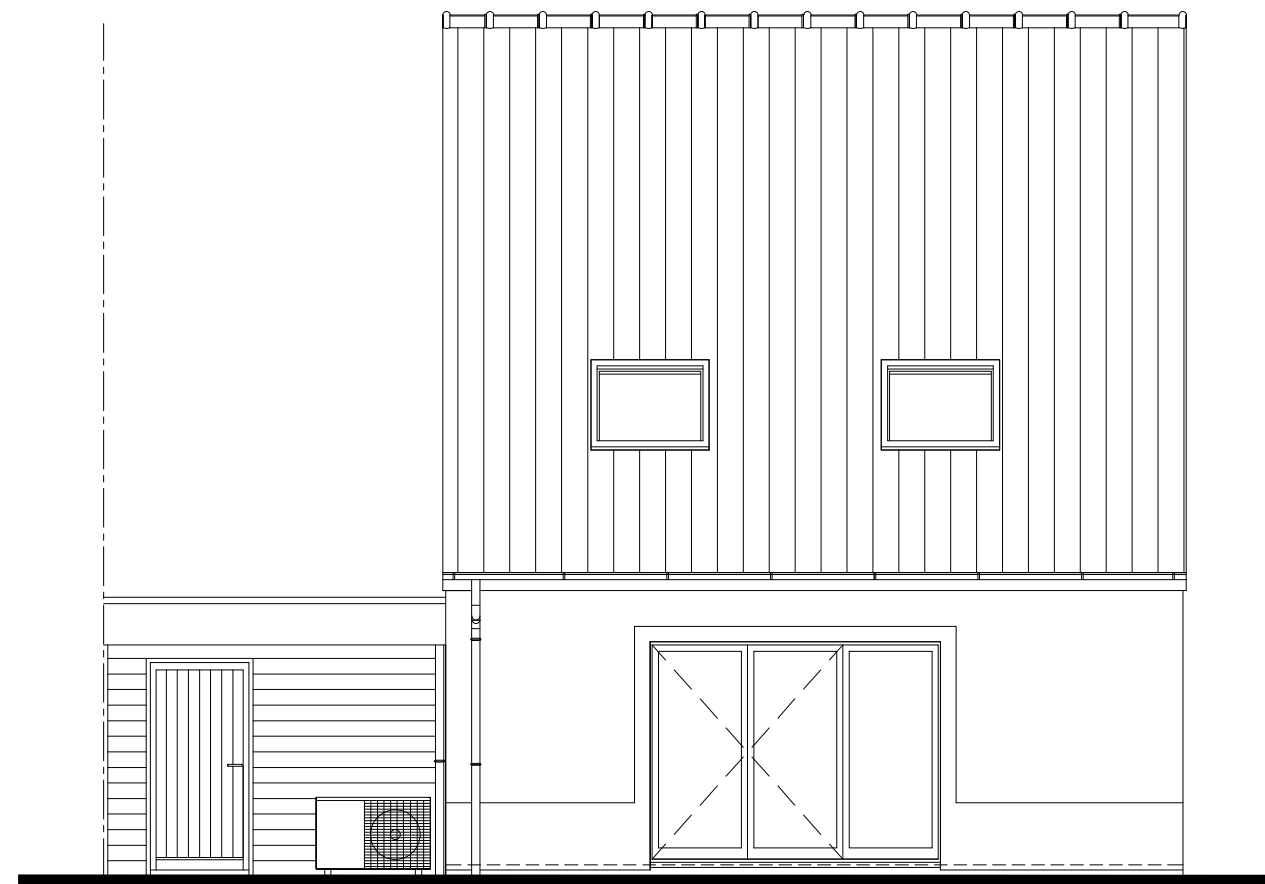
Elévation NORD
